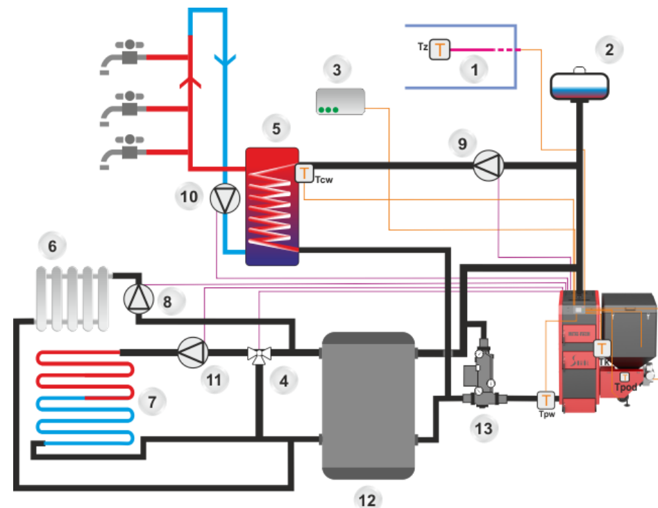
Rysunek 15.4 Podłączenie kotła do instalacji grzewczej z laddomatem i buforem
