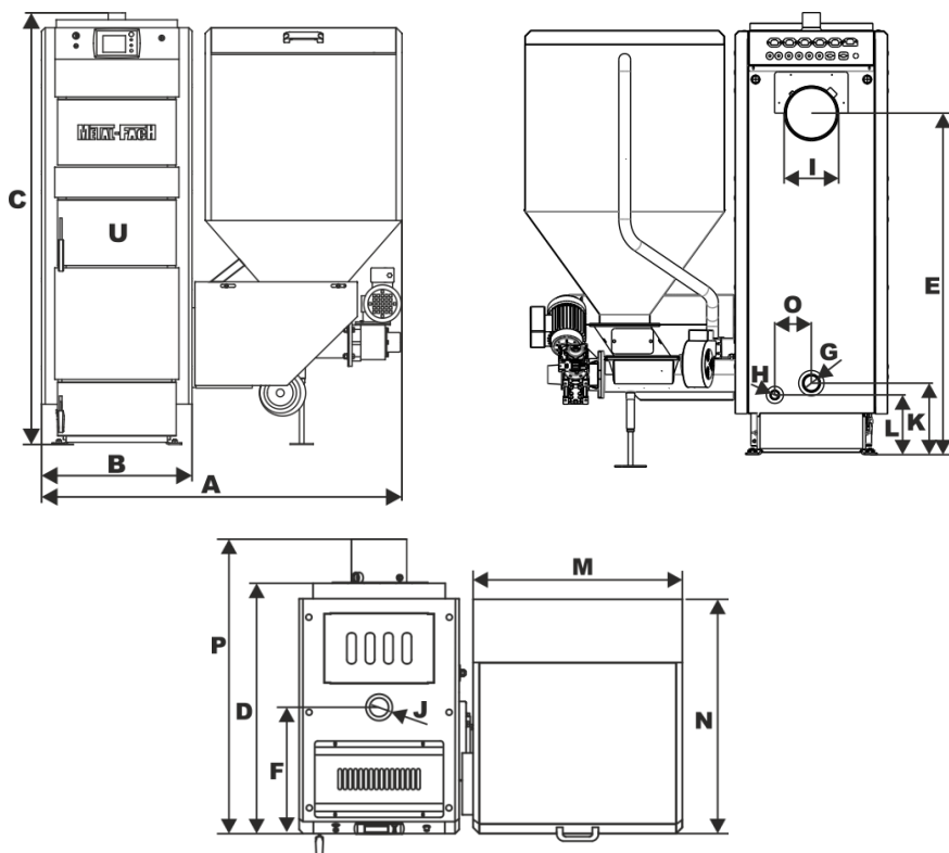
Rysunek 8.1 Wymiary kotła SEG/SEG PLUS
