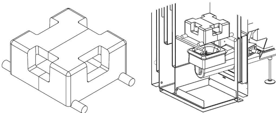
Rysunek 13.1 Ułożenie deflektora nad paleniskiem palnika.
