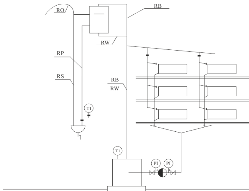
Rysunek 15.1 Schemat podłączenia kotła do instalacji grzewczej
