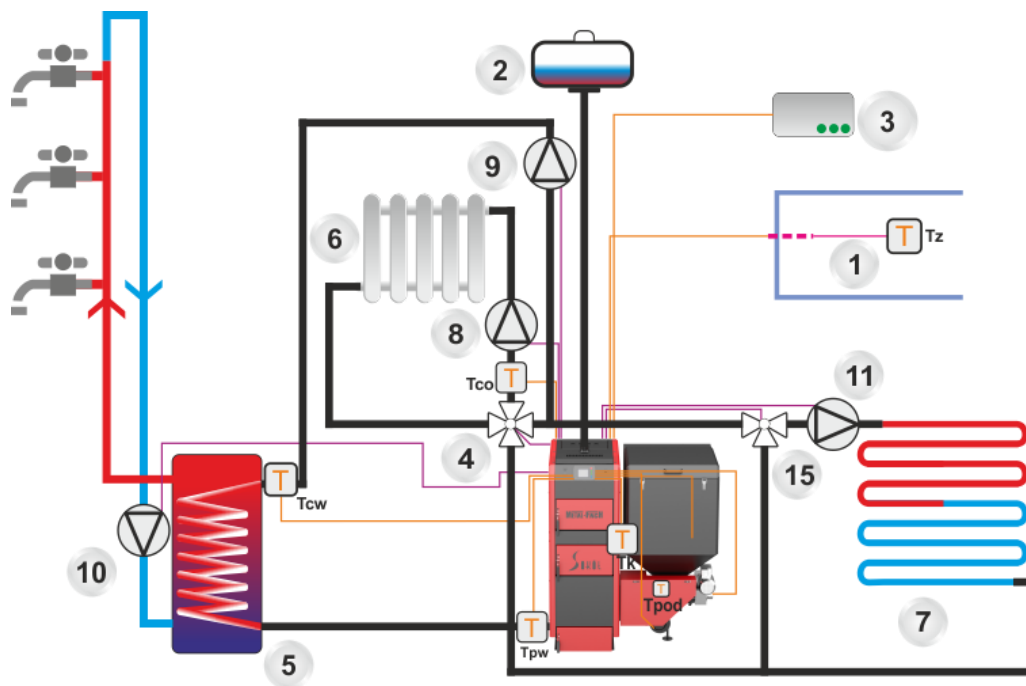
Rysunek 15.3 Podłączenie kotła do instalacji grzewczej
