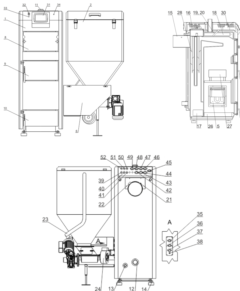
Rysunek 7.1 Podstawowe elementy budowy kotła SEG 14-38 kW
