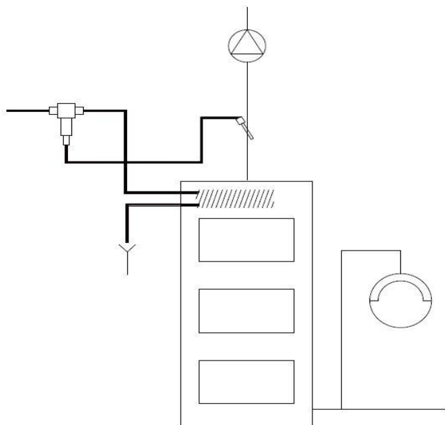
Rysunek 16.1 Schemat zabezpieczenia kotła za pomocą wbudowanej wężownicy chłodzącej i z zabezpieczeniem termicznym.
