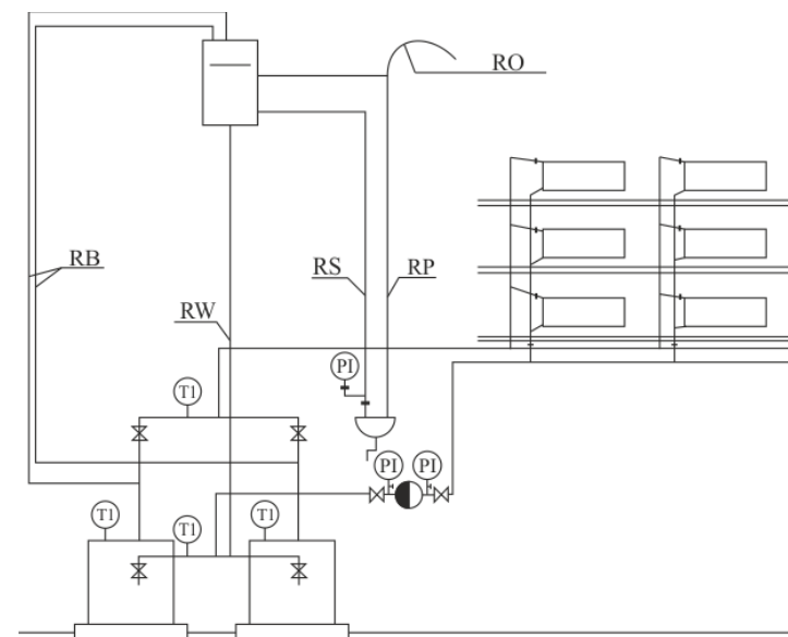
Rysunek 15.2 Schemat podłączenia kotła do instalacji grzewczej
