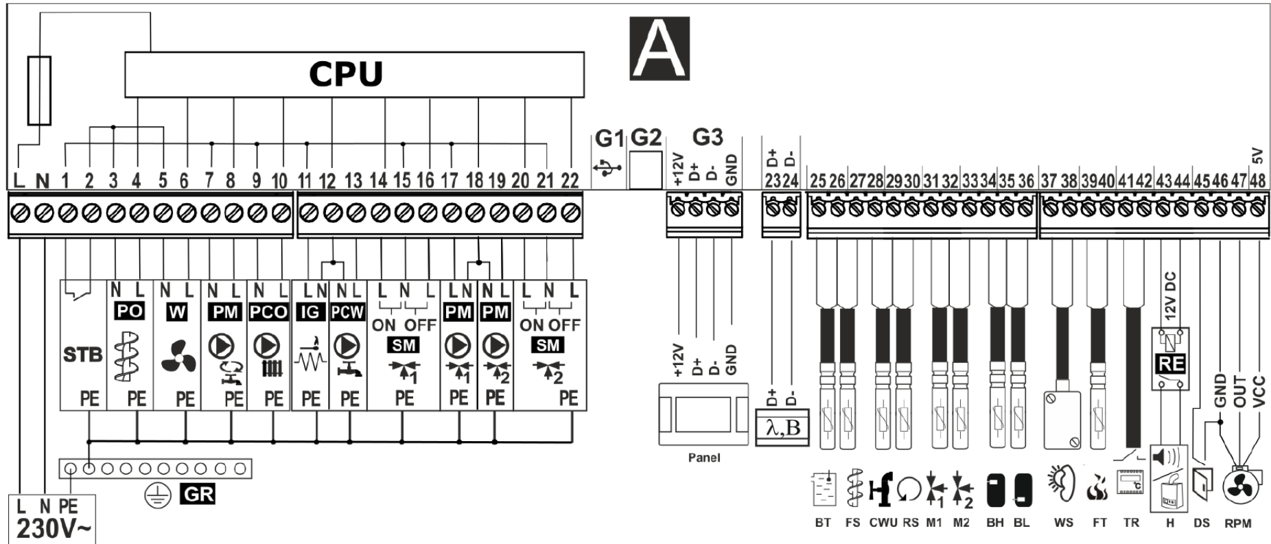
Rysunek 18.1 Schemat elektryczny podłączenia kotła - PLATINUM.
